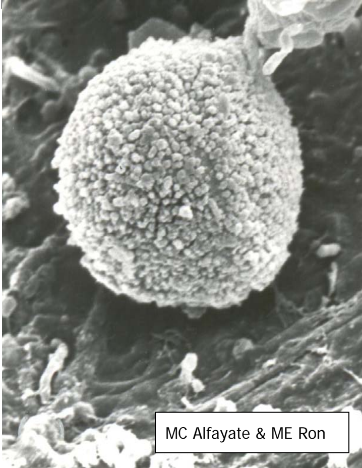
N. cephalonica
