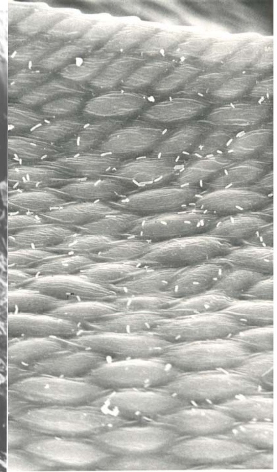
N. intermedia
